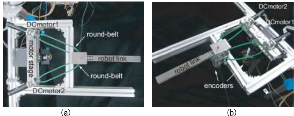
図1. 丸ベルトのねじりを利用した新アクチュエータの開発
